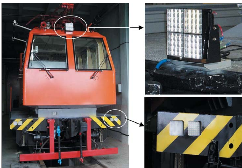
Рис. 3. Светодиодные светотехнические устройства буферной балки локомотива и лобовой прожектор
